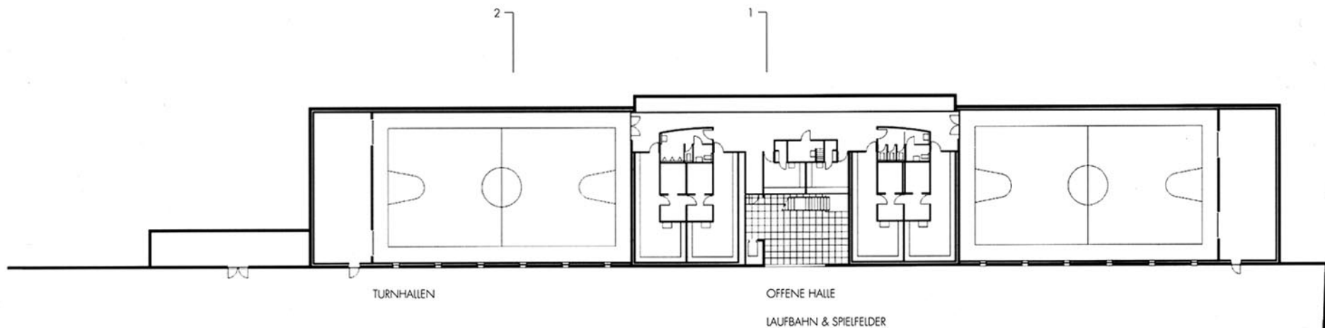
GRUNDRISS NIVEAU 1
