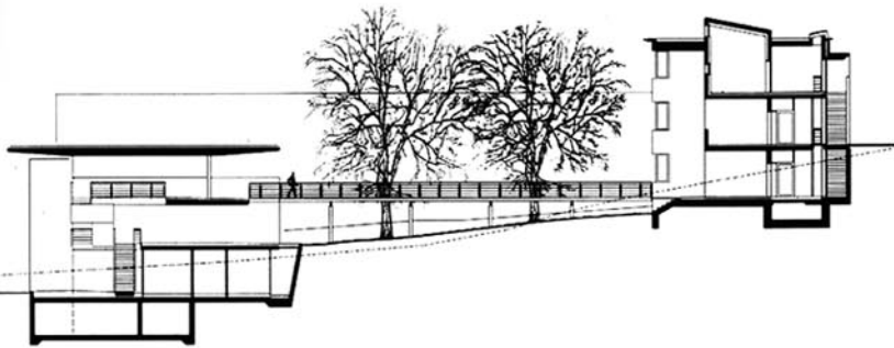
SCHNITT 1
