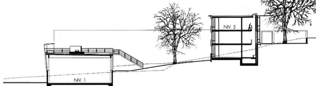
SCHNITT 2
