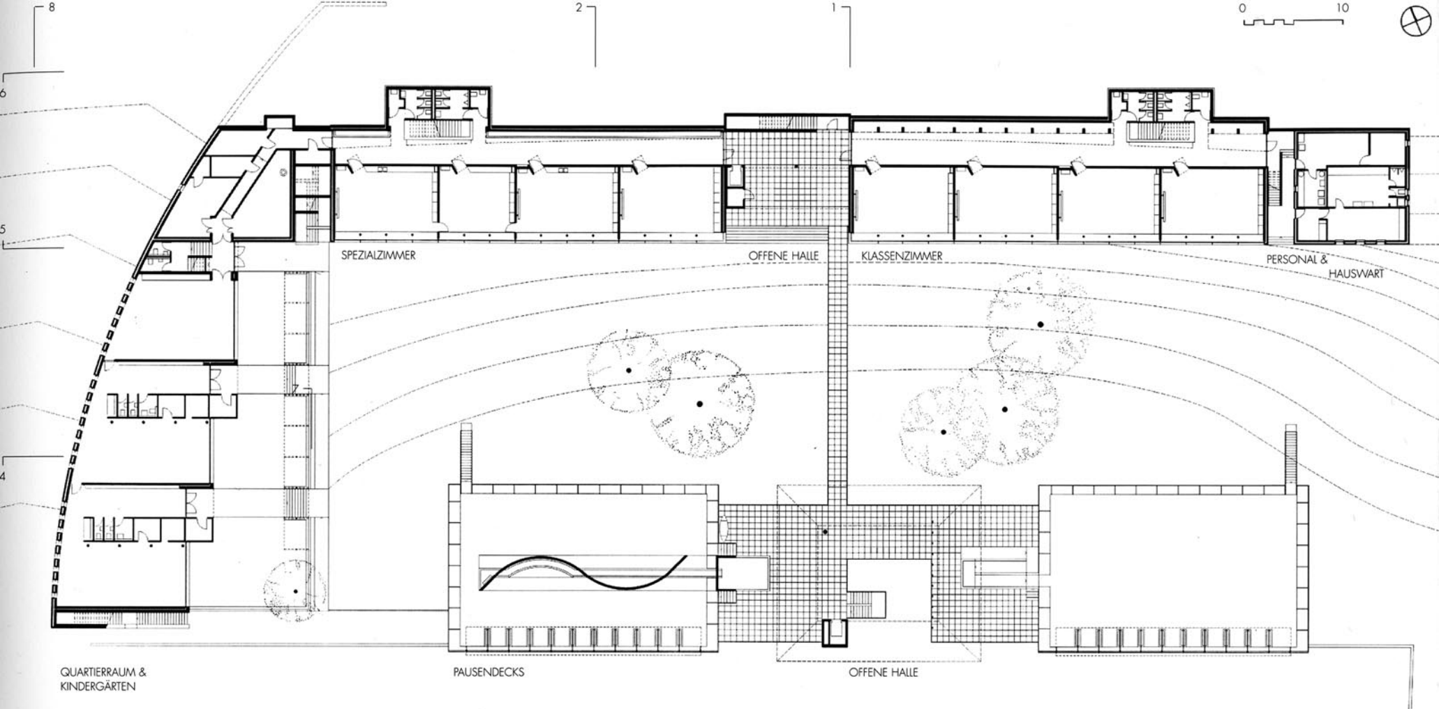
GRUNDRISS NIVEAU 3
